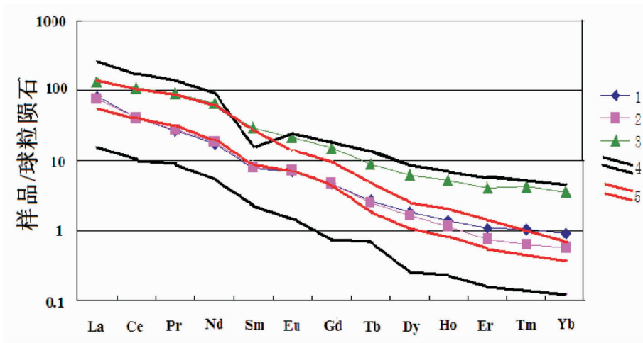
图 4 橄榄岩捕虏体全岩 REE 配分曲线
