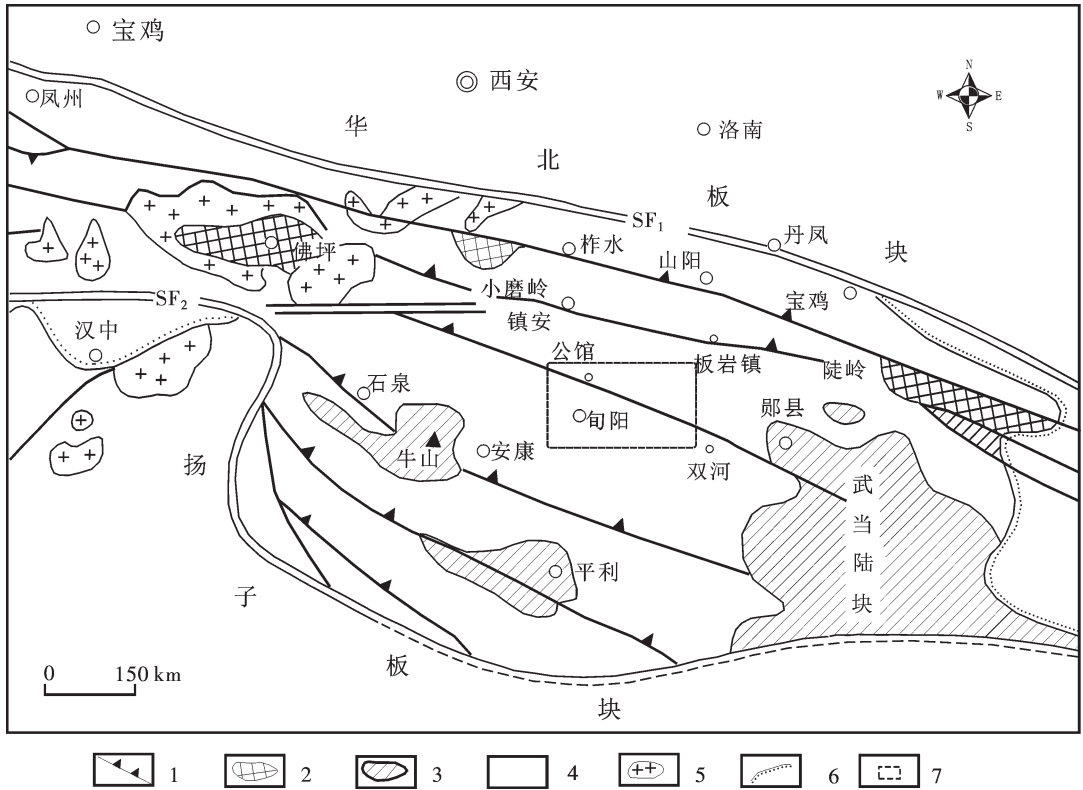
图1 南秦岭(东部)区域地质略图(据张国伟等 [14] ,2001 编绘)
