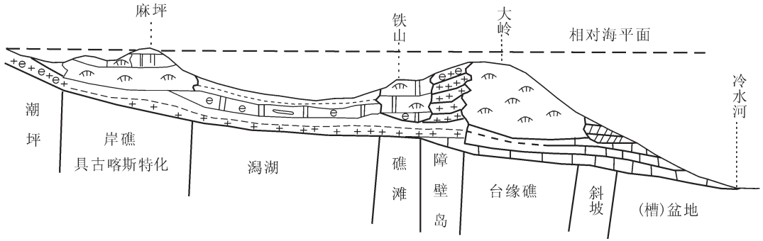
图2 中泥盆统石家沟组麻坪—冷水河一带沉积环境演化示意图
